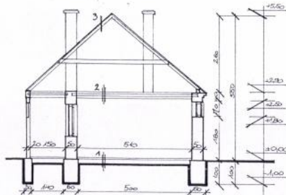
F-F METSZET M=1:100
