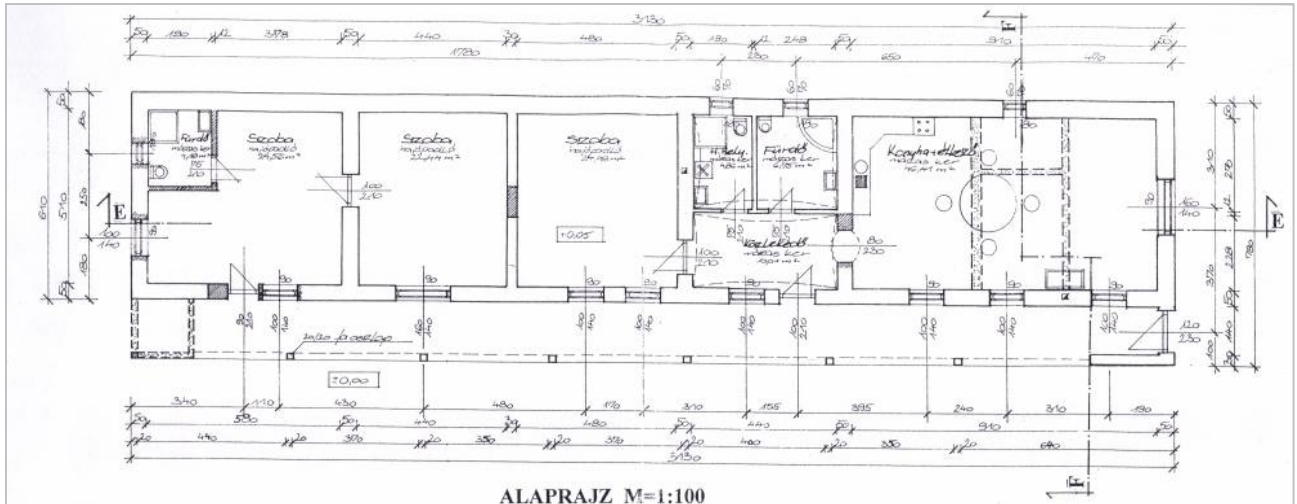
ALAPRAJZ M=1:100
